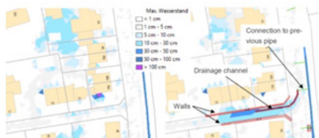
Análise de drenagem para Neugraben-Fischbek (© Hamburg Wasser)
