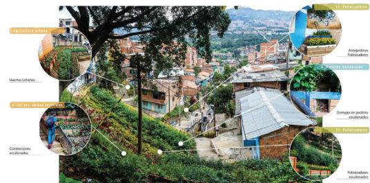
Intervenções iniciais na Quebrada Juan Bobo (© projeto Urban GreenUP)
