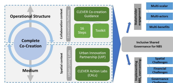
Figura: Conceito da cocriação completa para a implementação de SbN (Mahmoud & Morello, 2021)
